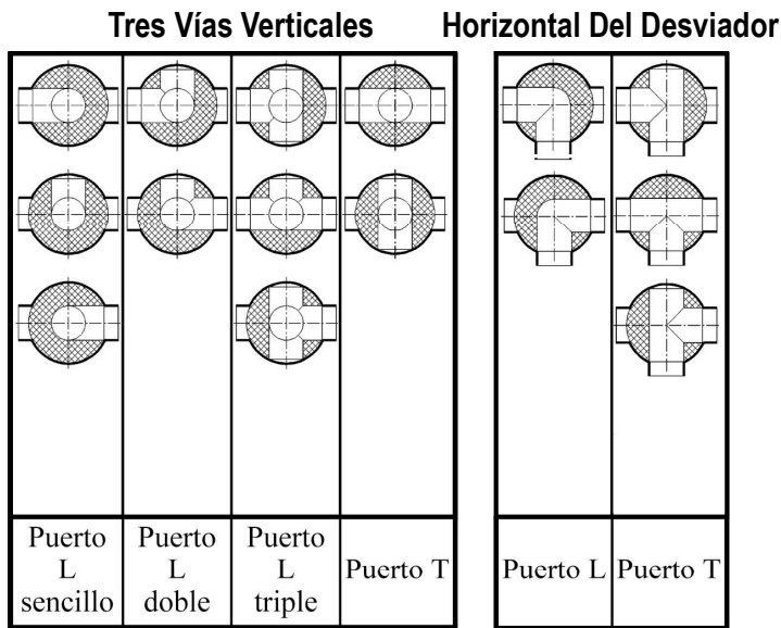
Opciones de Puerto de Bola Vistas Desde la Parte Superior de la Válvula
