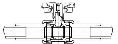
VALVULA DE BOLA TRUE UNION 2000 CON JUEGO DE RECONVERSION
